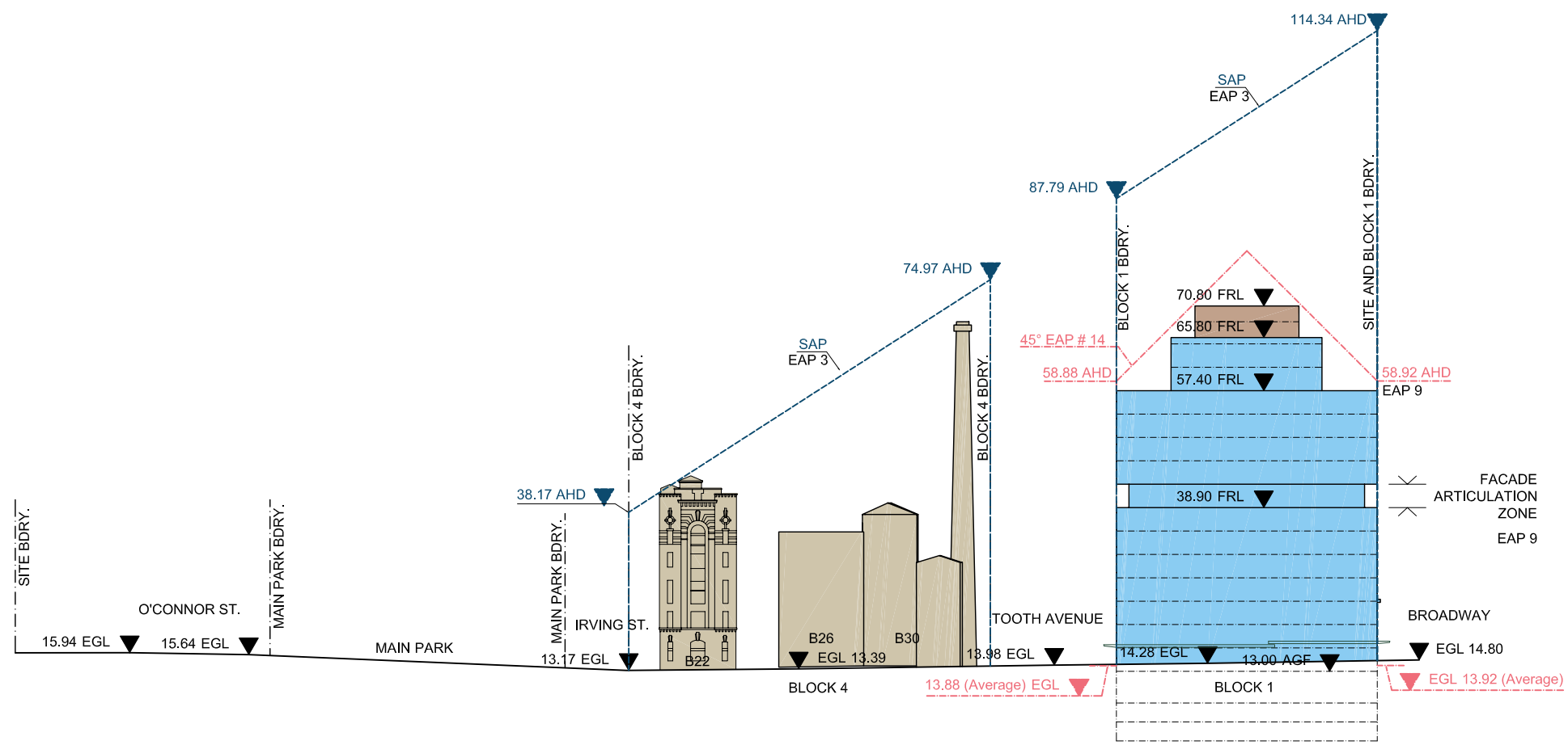
ELEVATION 04
